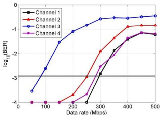
Рисунок 7. Скорость передачи данных в зависимости от BER для каналов МИМО.
